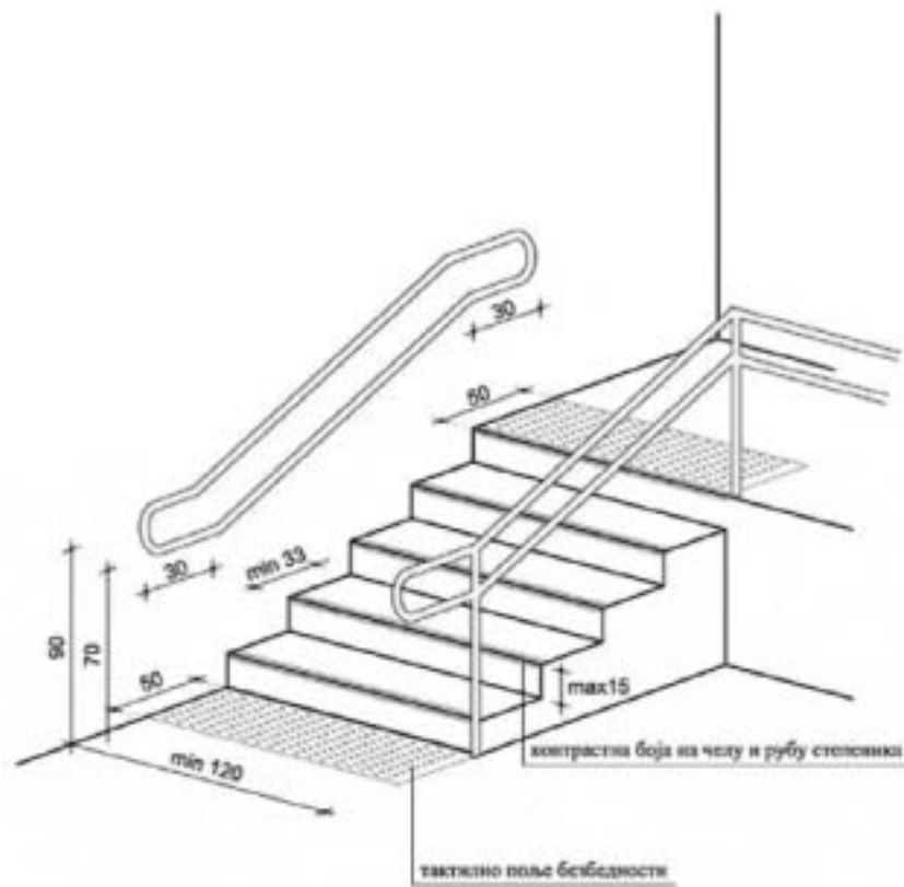
Слика 5. Ступенице и ступеништа
